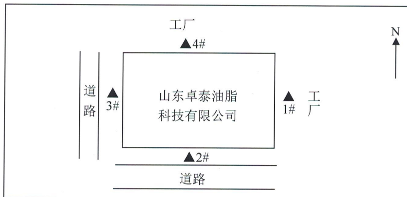
附图 1: 2022.04.22 山东卓泰油脂科技有限公司厂界噪声测点示意图
